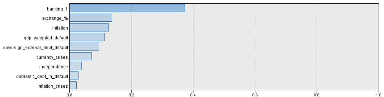
Рис. 5. Важливість предикатів нейронної мережі
