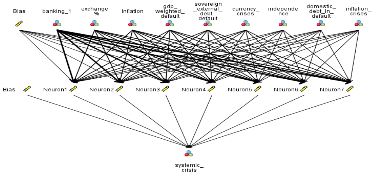
Рис. 4. Загальний вигляд нейронної мережі
