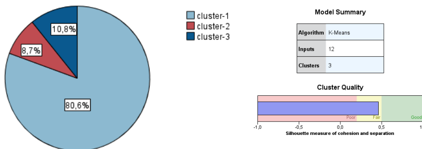
Рис. 2. Характеристика кластерів за K-means
